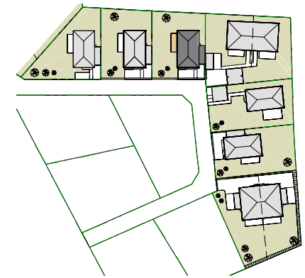
LAGEPLAN
