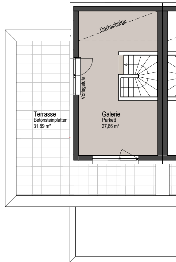
DACHGESCHOSS
