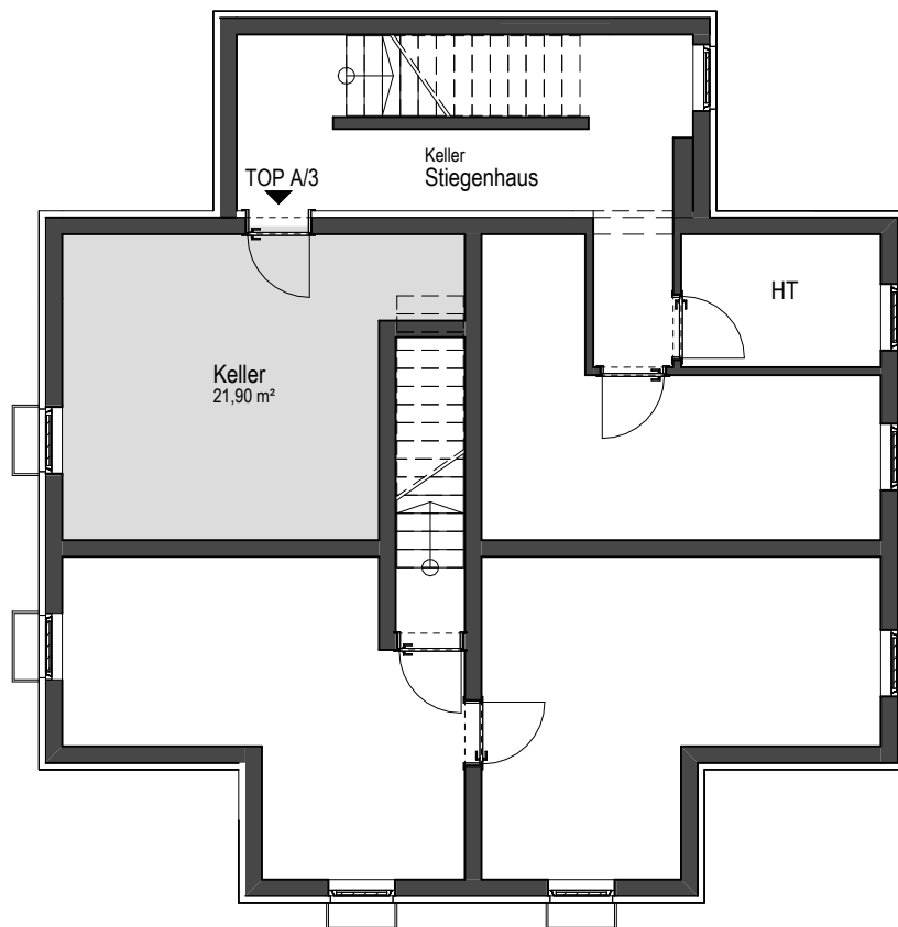
KELLERGESCHOSS
