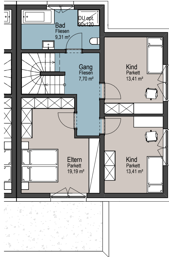
OBERGESCHOSS
