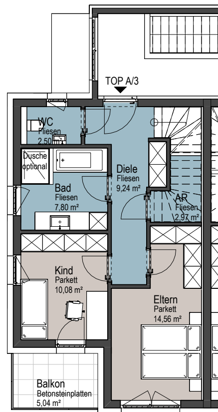
OBERGESCHOSS
